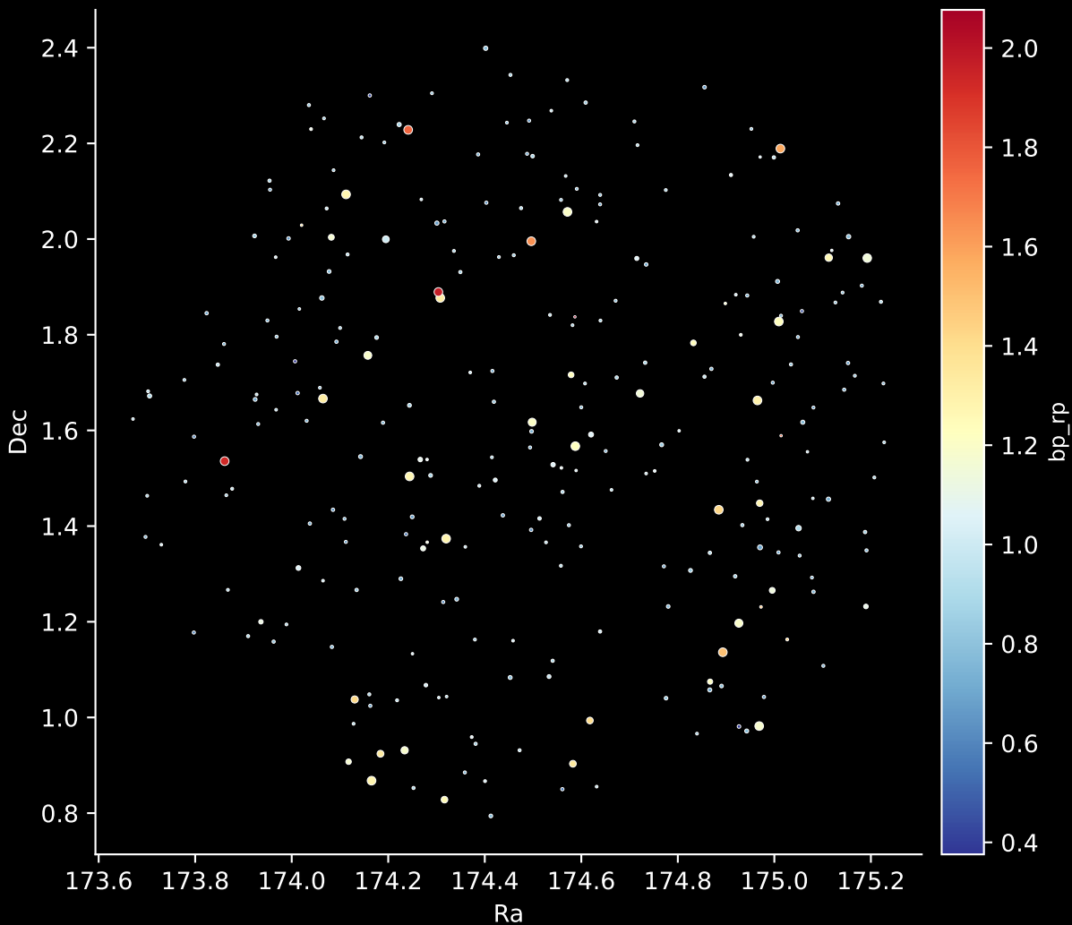
GALAH DR4 Field: [1598] Stars: 267
