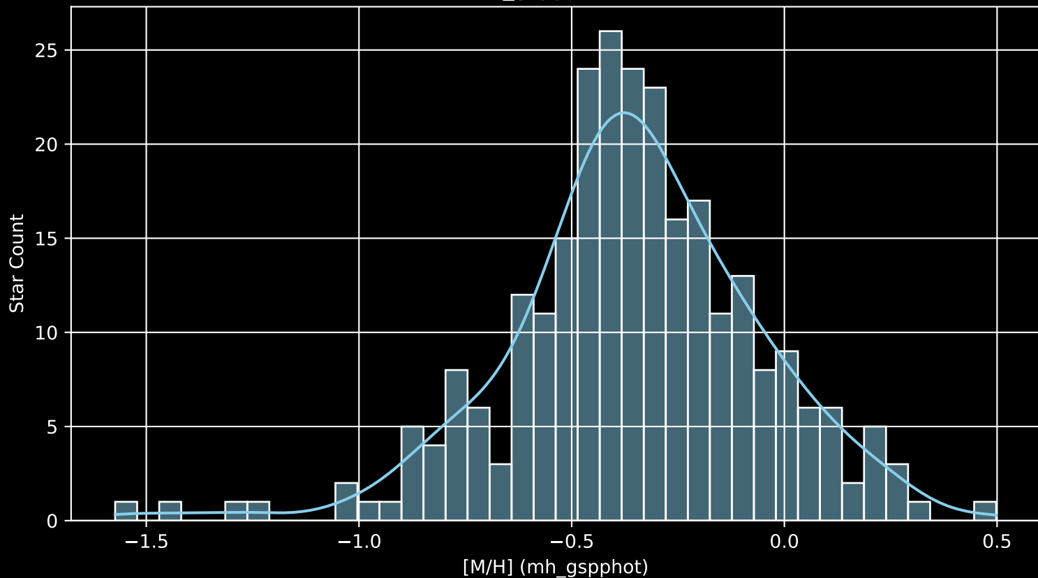
GALAH DR4 Field: [1598] [M/H] (mh_gspphot) (n= 267)
