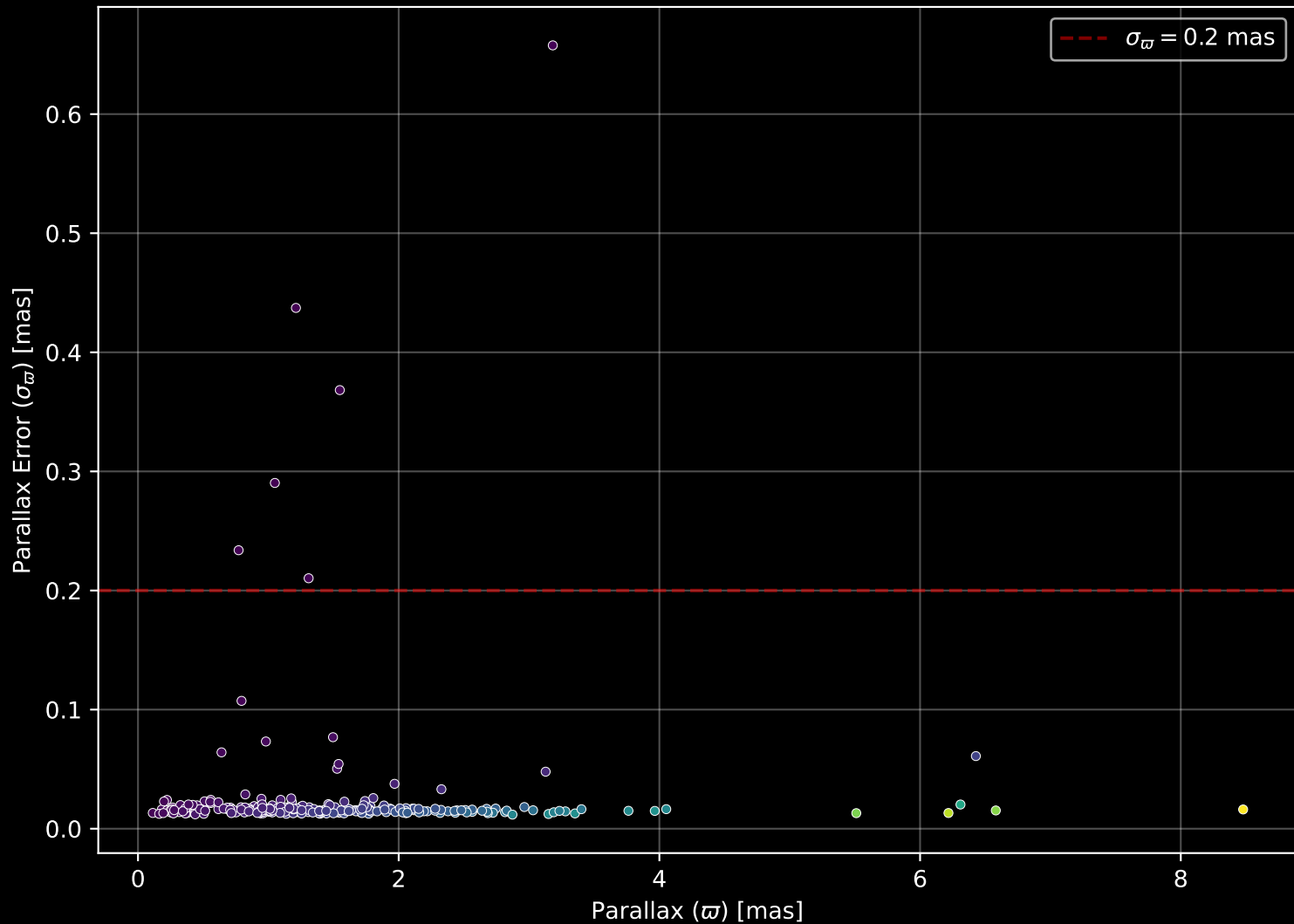
GALAH DR4 Field: [1598] Parallax Quality (n= 267)
