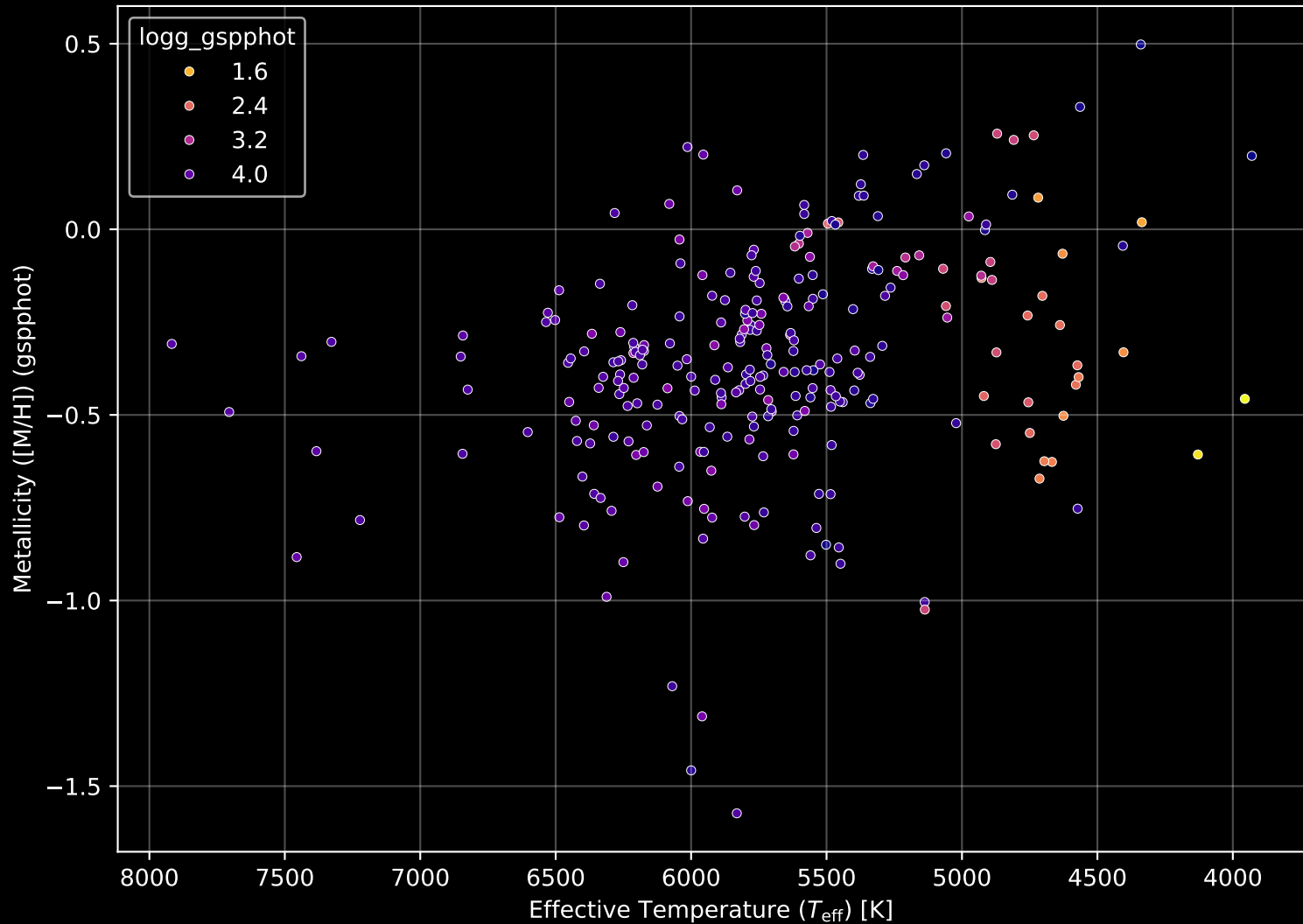
GALAH DR4 Field: [1598] Stellar Population Parameters (n= 267)
