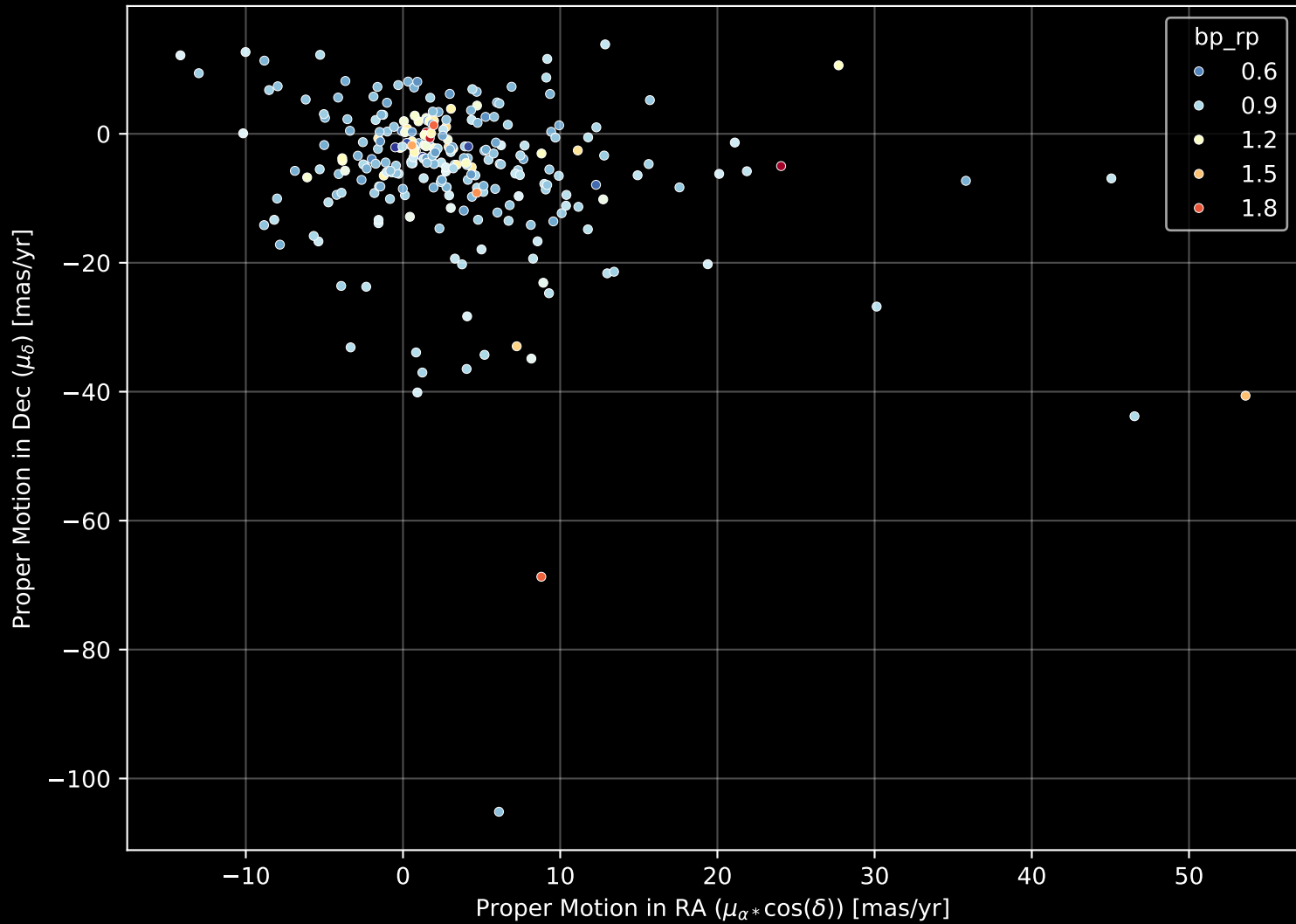
GALAH DR4 Field: [1598] Proper Motion Diagram (n= 267)
